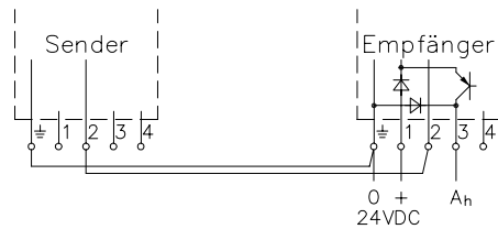
Anschlussplan
